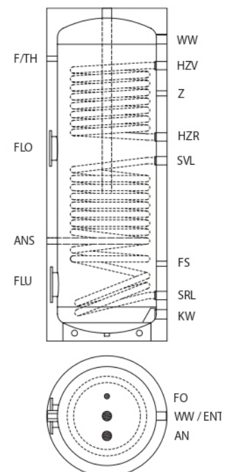
BRR 800 - 2000
