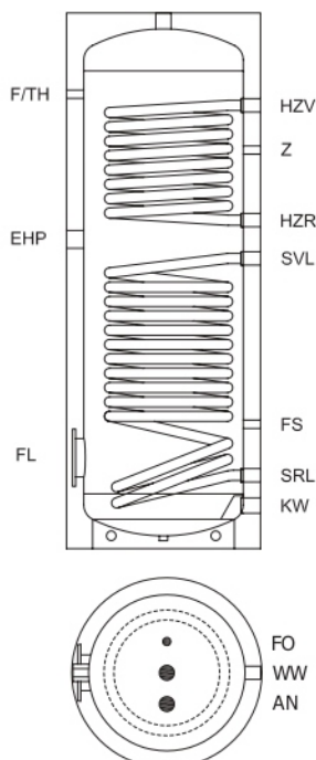
BRR 200 - 500
